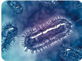
Escherichia Coli
